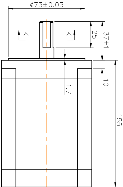
外型图:
